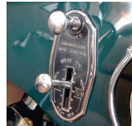
Ülal nn toore klapp, alumiselt kangilt saab reguleerida karburaatori õhuvõttu (soe või külm).
